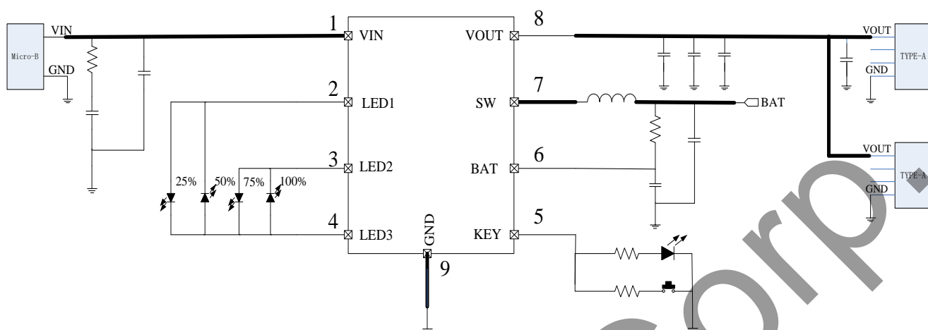
图 1 简化应用原理图
