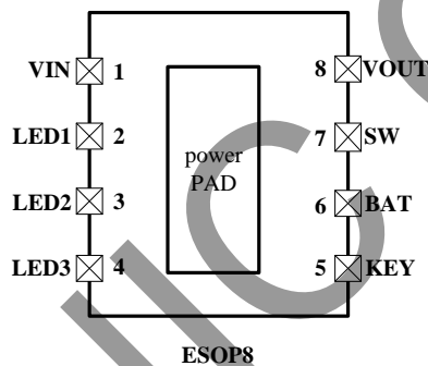
图 2 IP5306 引脚图
