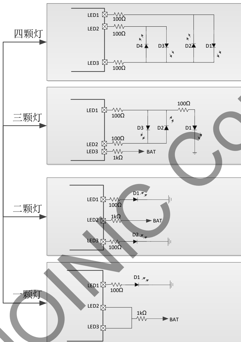
图 3 4、3、2、1 灯电路连接方式
