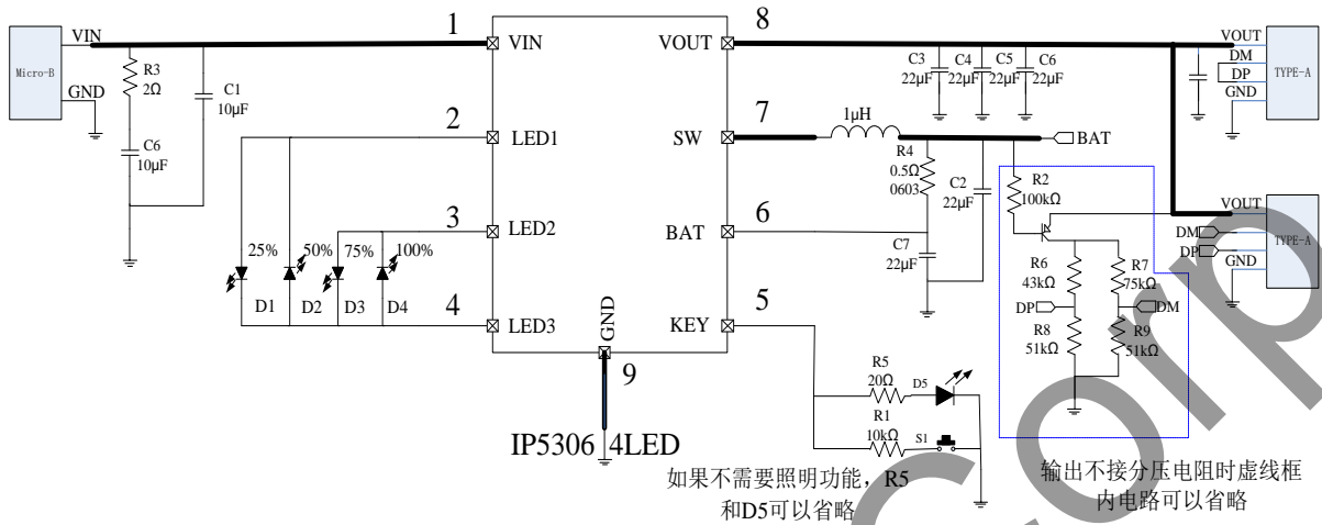
图 4 4LED 电量显示典型应用原理图
